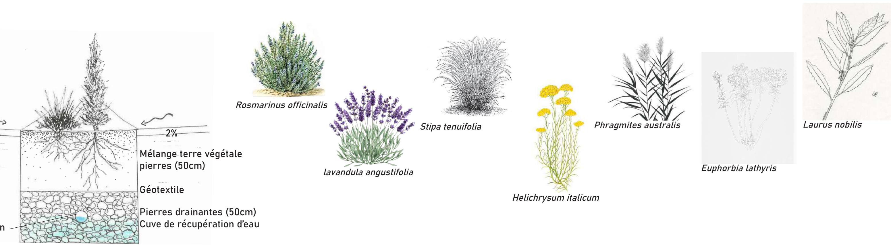
Coupe technique des massifs récupérateurs d'eau
