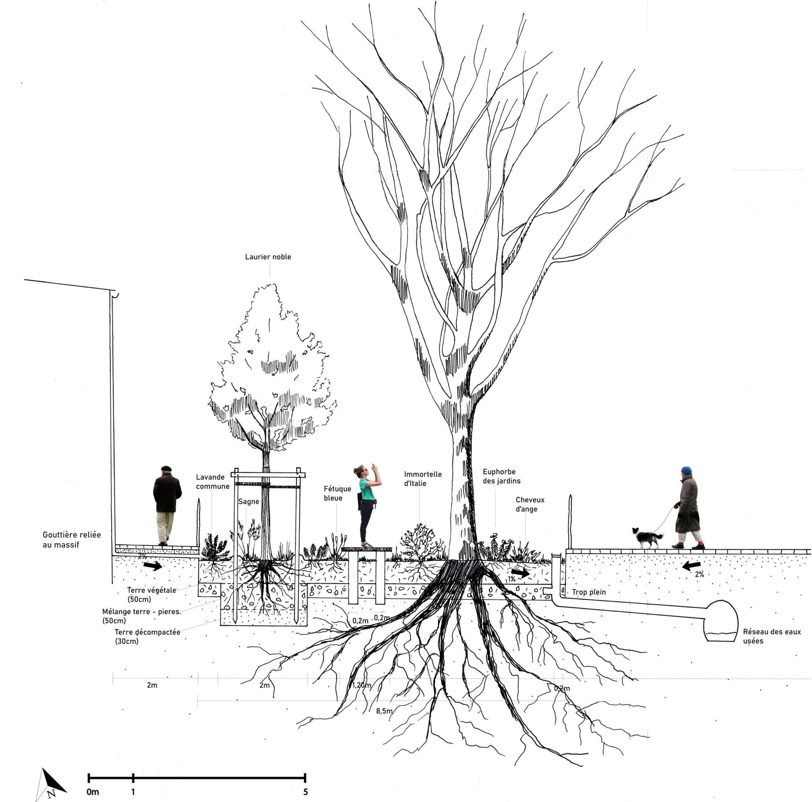
Coupe technique des massifs récupérateurs d'eau
